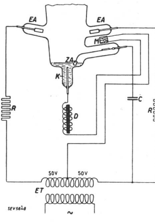
Fig. 2. Resonanzzündung.
