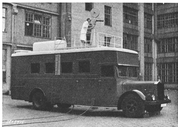
Fig. 1. Fernsehaufnahmewagen.
