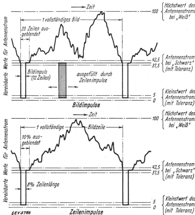
Fig. 1. Baird-System.
