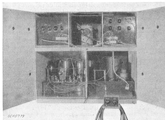
Fig. 5. Telefunken-Grossbildempfänger von hinten. Die Kathodenstrahlröhre befindet sich im mittleren Fach oben.
