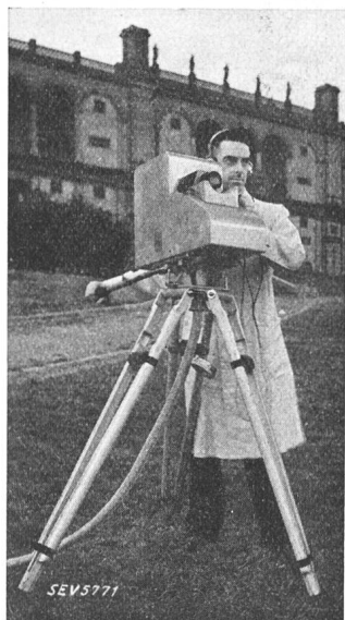
Fig. 5. Emitron-Kamera.
