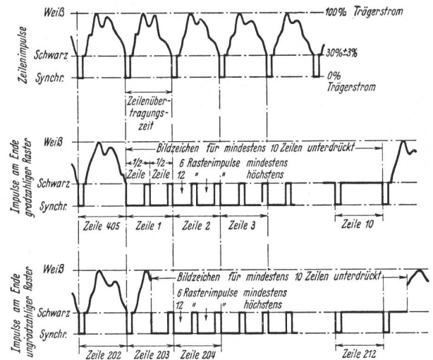
Fig. 2. Marconi-EMI-System.
