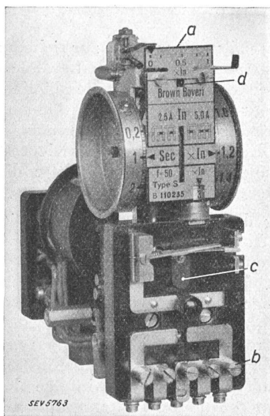
Fig. 3. Stromanzeigendes Sekundärrelais (ohne Verschaltung). a Betriebsstrom- anzeige. b Umschalt- und Prüfklappen. c Kontaktsignal. d Anlaufanzeiger.
