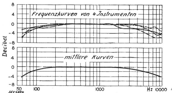
Fig. 5. Frequenzkurven von Band-Mikrophonen.
