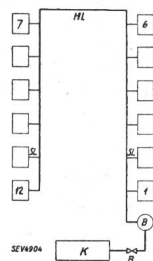
Fig. 10. Druckluftversorgung von 12 installierten Druckluftschnellschaltern.
