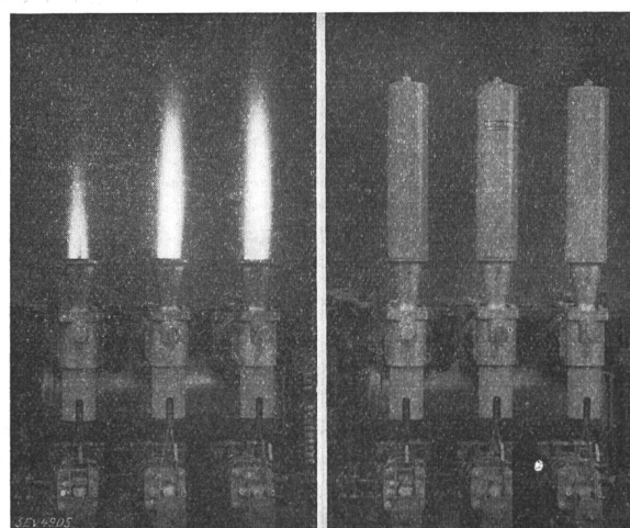
Fig. 11. Aeusserer Erscheinung an einem 100 MVA-Druckluftschnell-schalter, links ohne, rechts mit aufgesetzten Auspuffkühlern. Eff. Abschaltstrom in beiden Fällen 10 000 A. Die Ungleich-heiten an den drei Polen sind auf verschiedene Phasenlage des Stromes im Augenblick der Kontakttrennung zurückzuführen.
