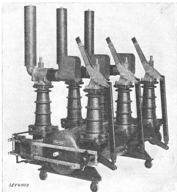
Fig. 9. Druckluftschnellschalter in liegender Anordnung. Nennspannung 50 kV; Abschaltleistung 600 MVA.
