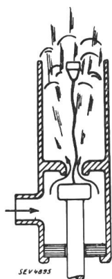
Fig. 1. Kontaktanordnung mit allseitiger Luft- bebläsung des Lichtbogens.
