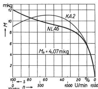
Fig. 34. 4 poliger Drehstrom-Asynchronmotor, 8 PS, mit nutenlosem, radial geschichtetem Anker (NLA 6) nach Fig. 21 a und mit Käfiganker (KA 2) von gleichem Nennschlupf 50 Per./s, U_1 \approx 330 V \Upsilon Verlauf des Drehmomentes M mit der Drehzahl n . D_r = 199,2 mm \varnothing , l_1 = 85 mm.
