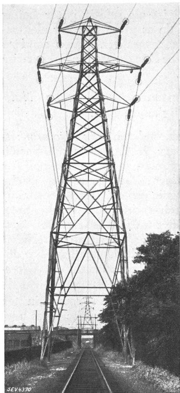
Fig. 4. «Grid»-Primärleitung längs Bahntracé. (Photo CEB.)
