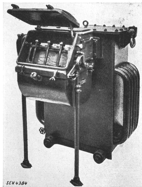
Fig. 17. Transformator, mit Schalter und Sicherungen zusammengebaut. Der Schalterdeckel kann nur bei ausgeschaltetem Schalter geöffnet werden; die Sicherungen können von Hand ersetzt werden, da das Schalterinnere durch Isolierplatte abgedeckt ist. (Brush, Ltd. Longborough.)
