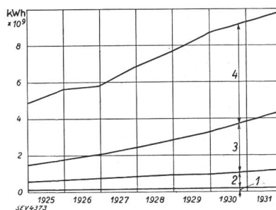
Fig. 6. Energieabgabe in den Jahren 1925 bis 1931. 1 für öffentliche Be- leuchtung. 2 für Bahnbetrieb. 3 für Beleuchtung u. Haushalt. 4 für Motoren.
