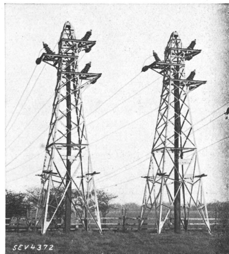
Fig. 5 b. 33 kV «Grid»-Sekundärleitungen. Kabel-Endmasten. (Photo CEB.)
