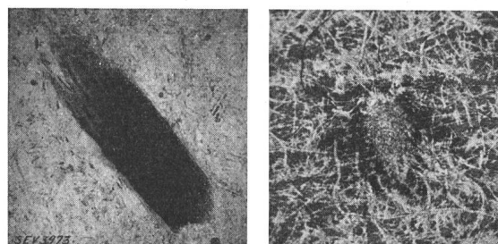
Faserknoten aus nicht gleichmässig verteilten Fasern.
