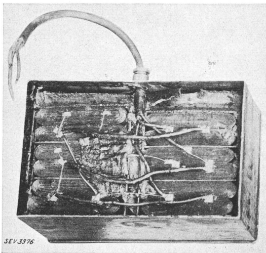
Fig. 10. Kleiner Kondensator mit Flachwickeln in Masse.
