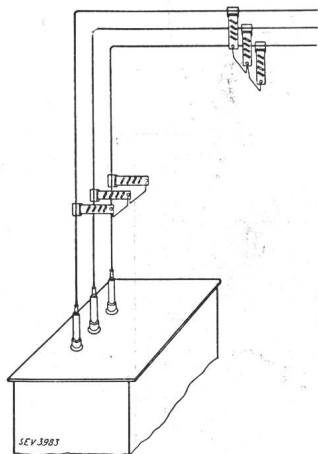
Fig. 19. Hochspannungs- Entladewiderstände.
