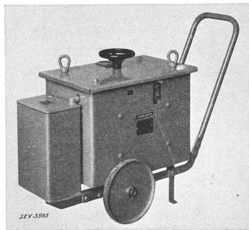
Fig. 21. Schweißapparat mit angebautem Kondensator.
