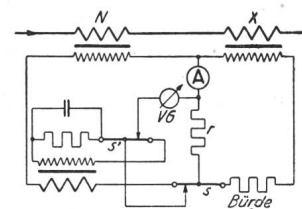
Fig. 4. Ausgeführte Prüf- schaltung.
