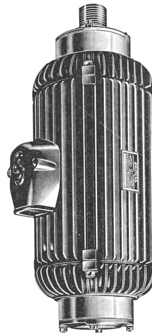
Fig. 6. Fräsmotor mit Einspannhalsen 1,8 kW; 8600 U/min.
