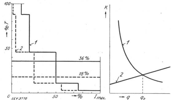
Fig. 3. Jahresbelastungsdiagramm einer Anlage mit 3160 «Benutzungsstunden» bei 1580 «Verluststunden» ( f_v = 18\% ). 1 Belastungsdiagramm. 2 Verlustdiagramm (Maßstab 100 mal kleiner).
