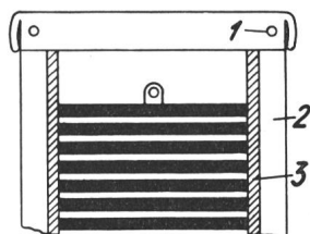
Fig. 2 (rechts). Einfassung der Heizplatten. 1 Bolzen, 2 Einfassung, 3 Isolation.
