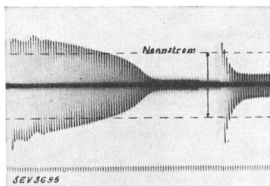
Fig. 6. Leeranlauf gegen kleine Schwungmassen. Einschaltstromstoss \approx 1,6 \cdot Nennstrom. Umschaltstromstoss \approx 1,5 \cdot Nennstrom.
