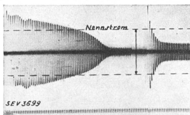
Fig. 7. Leeranlauf gegen kleine Schwungmassen. Einschaltstromstoss \approx 1,6 \cdot Nennstrom. Umschaltstromstoss \approx 1,5 \cdot Nennstrom.
