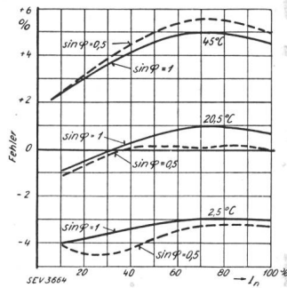
Fig. 4. Dreiphasenblindverbrauchzähler.
