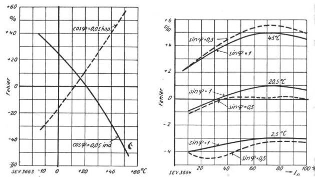
Fig. 3. Dreiphasenzähler Fabrikat A.
