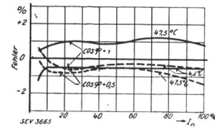
Fig. 5 (oben). Dreiphasenpräzisionszähler.
