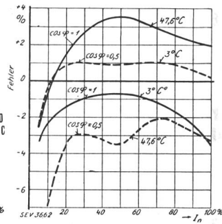
Fig. 2. Dreiphasenzähler Fabrikat B.
