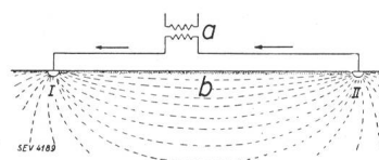
Fig. 1. Prinzipisches Schema für die Wirkungsweise einer Erdung. a Stromquelle b Erde I Elektrode I II Elektrode II
