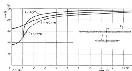
Fig. 10. Spannung in % der an der Erdung liegenden Spannung an der Erdoberfläche für verschieden tief eingegrabene, horizontal verlegte Rohrelektroden, in der Axenrichtung der Elektrode gemessen.
