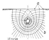
Fig. 8. Eingegrabene Kugelelektrode. a Spannungskurven. b Stromlinien.
