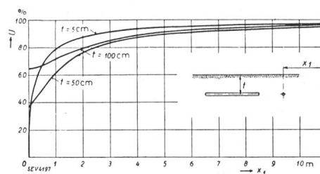
Fig. 9. Spannung in % der an der Erdung liegenden Spannung an der Erdoberfläche für verschieden tief eingegrabene, horizontal verlegte Rohrelektroden, senkrecht zur Elektrodenaxe gemessen.
