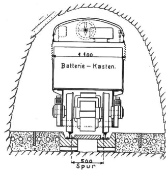
Kraftwerke Oberhasli A.G. Stollenbahn Handeck-Guttannen. Akkumulatoren-Lokomotive.
