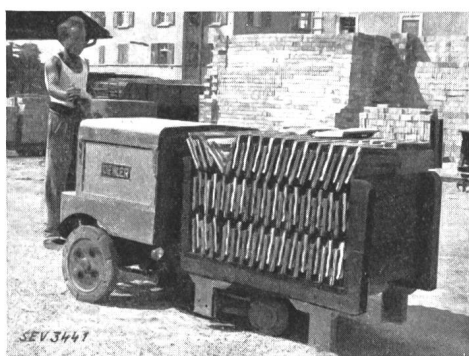
Fig. 7. Hubkarren beim Ziegeltransport, 1 1/2 t.
