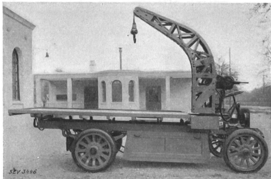
Fig. 2. Lastwagen mit Kranaufbau. Nutzlast 5 t, Kran 2 t.
