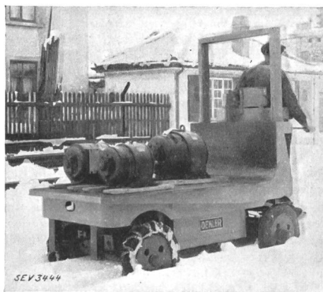
Fig. 5. Stapelkarren im Schnee, 2 t. Hubhöhe 2,5 m.
