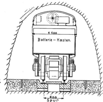
Kraftwerke Oberhasli A.-G. Stollenbahn Handeck-Guttannen. Akkumulatoren-Lokomotive.
