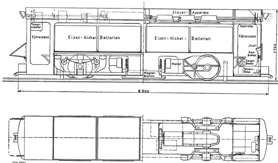
Kraftwerke Oberhasli A.G. Stollenbahn Handeck-Guttannen. Akkumulatoren-Lokomotive.
