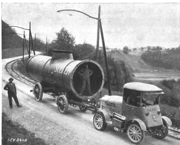
Fig. 3. Akkumulatortraktor. Zugkraft 10 t.
