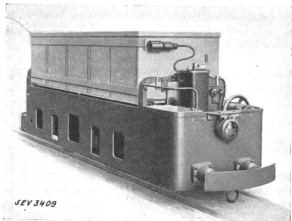
Fig. 7. Akkumulator-Grubenlokomotive mit Abrollvorrichtung zur Auswechslung der Batterie.
