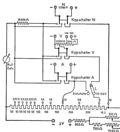
Fig. 1. Schaltbild.
