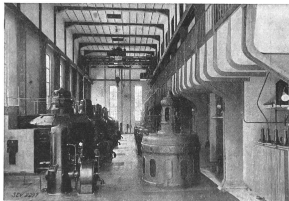
Fig. 2. Maschinenraum Rempen; links Generator-, rechts Pumpengruppe. (Aus Bull. SEV 1932, Nr. 2.)
