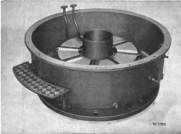
Fig. 6. EWC-Spurlager, geöffnet, mit unterem Spurring.
