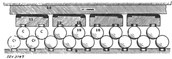
Fig. 12. Konstruktive Ausführung der Segmentlagerung auf Kugeln.
