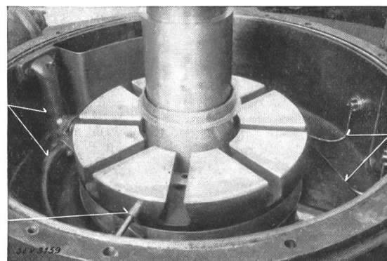
Fig. 4. EWC-Spurlager im Lagerkübel.
