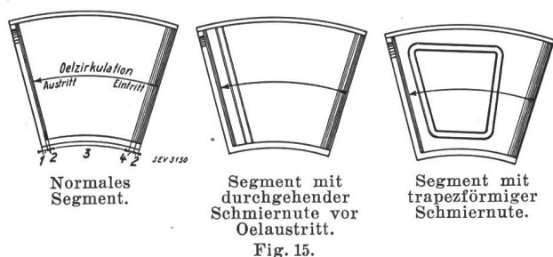
Versuche beim Auslauf und Stillstand der Maschine das Oel im Segmentinnern zurückzuhalten (Generatoren Rempen). 1 Öelkanal. 2 Abrundung. 3 Tragfläche. 4 Anzugfläche.
