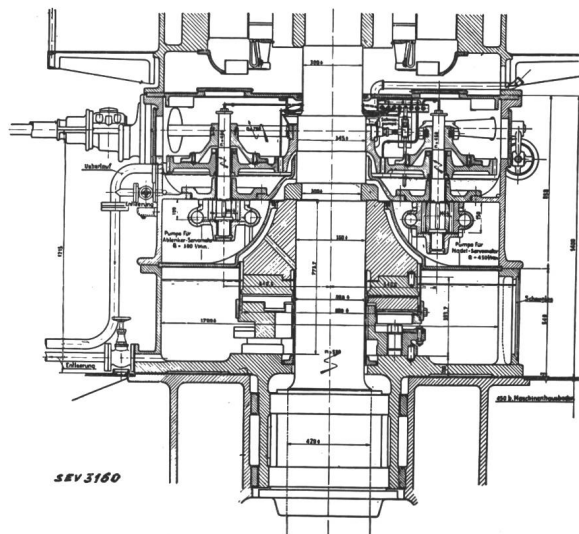
Fig. 5. Schnitt durch ein Kingsbury-Spurlager.
