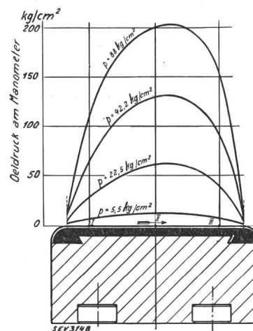
Fig. 13. Druckverteilung in der Umfangsrichtung eines Tragssegmentes bei verschiedenen Belastungen, gemessen an einem Versuchslager von Bell & Co.
