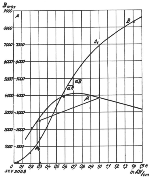
Fig. 6. Magnetisierungskurven für hochlegiertes Transformatorblech.
