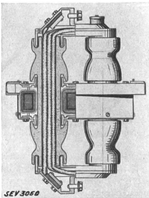
Fig. 7. Mehrleiter-Durchführungs- stromwandler, Form DS.
