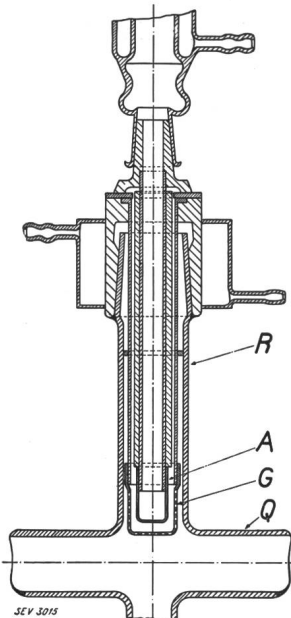
Fig. 1. Schnitt durch Anode und Gitter des Steuereinsatzes.
