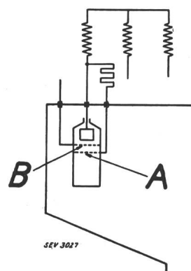
Fig. 13. Anode mit Erreger-, bzw. Ableiter- und Löschgitter.
