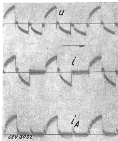
Fig. 14. Oszillogramm der Unterbrechung eines Gleichstromes.
