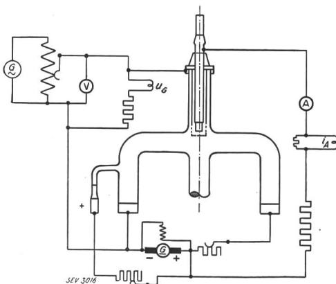
Fig. 2. Schaltschema.
