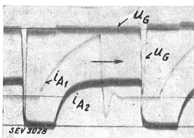
Fig. 14. Oszillogramm der Unterbrechung eines Gleichstromes.
