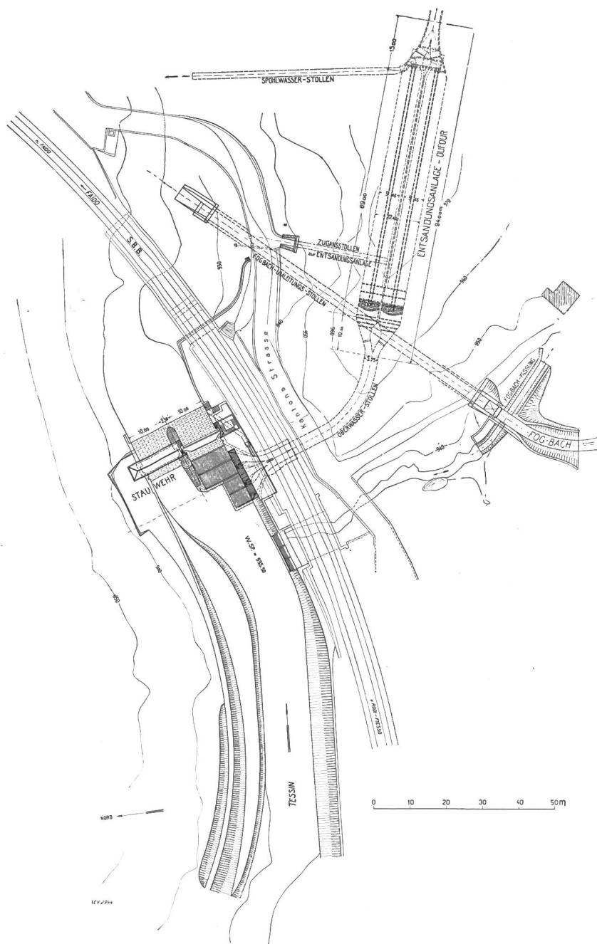
Fig. 2. Kraftwerk Piottino. Wasserefassung bei Rodi. Situation 1:1500.
