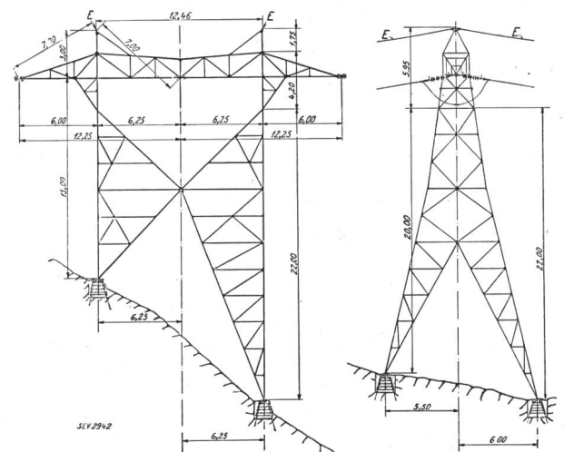
Fig. 18. Gotthardleitung Lavorgo-Amsteg. Abspannmast bis 1480 m Spannweite.
