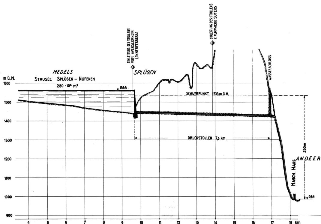
Fig. 2 (linke Hälfte). Projekt für die Ausnutzung der Hinterrhein-Wasserkräfte. Gefällstufe Splügen—Andeer. Maßstab: Horizontal 1 : 375 000; Vertikal 1 : 37 500.
