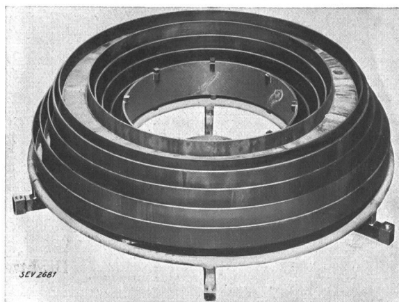
Fig. 11. Winkelringe, ineinandergestellt.
