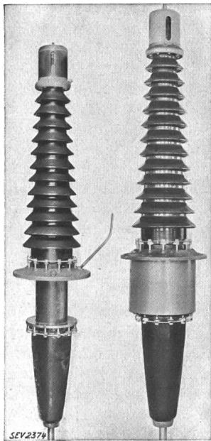
Fig. 4. Oelschalterdurchführungen der Micafil A.-G., ölgefüllt, für 150 kV Nennspannung, links ohne, rechts mit Stromwandler.
