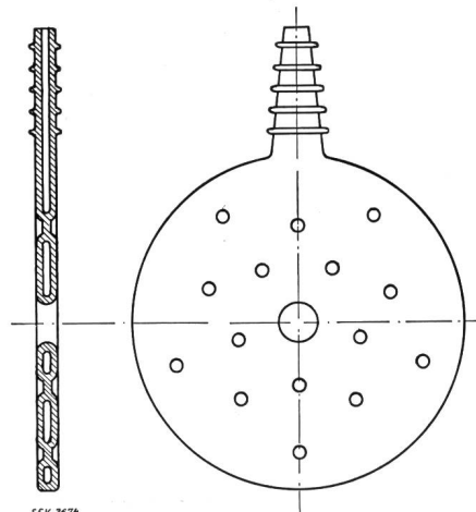
Fig. 2. Kopplungskondensator der Porzellanfabrik Rosenthal. Der eine Kondensatorbelag befindet sich in den Hohlräumen des Körpers mit Zuleitung durch den rohrähnlichen Ansatz; der andere befindet sich auf der äusseren Oberfläche, mit Zuleitung mittels eines Schraubenbolzens durch die Öffnung im Zentrum.
