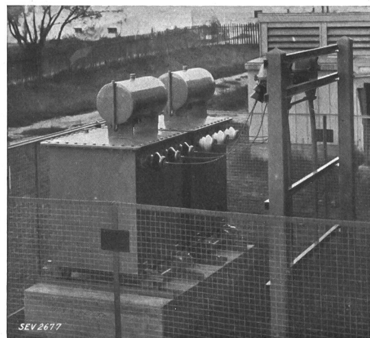
Fig. 6. Hochspannungskondensatoranlage der Micafil A.-G., 580 kVAr, 8000 V.
