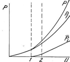
Fig. 2b. Verluste im Kabel in Funktion der Gesamtspannung (zwischen Seele und Mantel). P_i In den Luftfeinschlüssen. P_f Im festen Dielektrikum. P Gesamtverluste. Maßstäbe in linearer Teilung.
