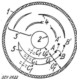
Fig. 1. Kabelquerschnitt mit Luftfeinschlüssen 1 Mantel. 2 Seele. 3 Festes Dielektrikum. 4 Luftfeinschlüsse Uebertrieben 5 Luftfeinschluss gross gezeichnet
