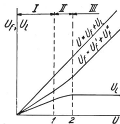
Fig. 2a. Spannungverteilung auf die Luftstrecke ( U_i ) und auf das feste Dielektrikum ( U_f ) bei ansteigender Gesamtspannung ( U ) (zwischen Seele und Mantel) vor und nach Eintritt des Glimmens.
