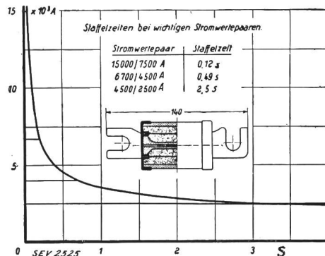
Fig. 1. Geschlossene Maschennetz-Sicherung, Bauart BEWAG. Strom-Zeit-Charakteristik.
