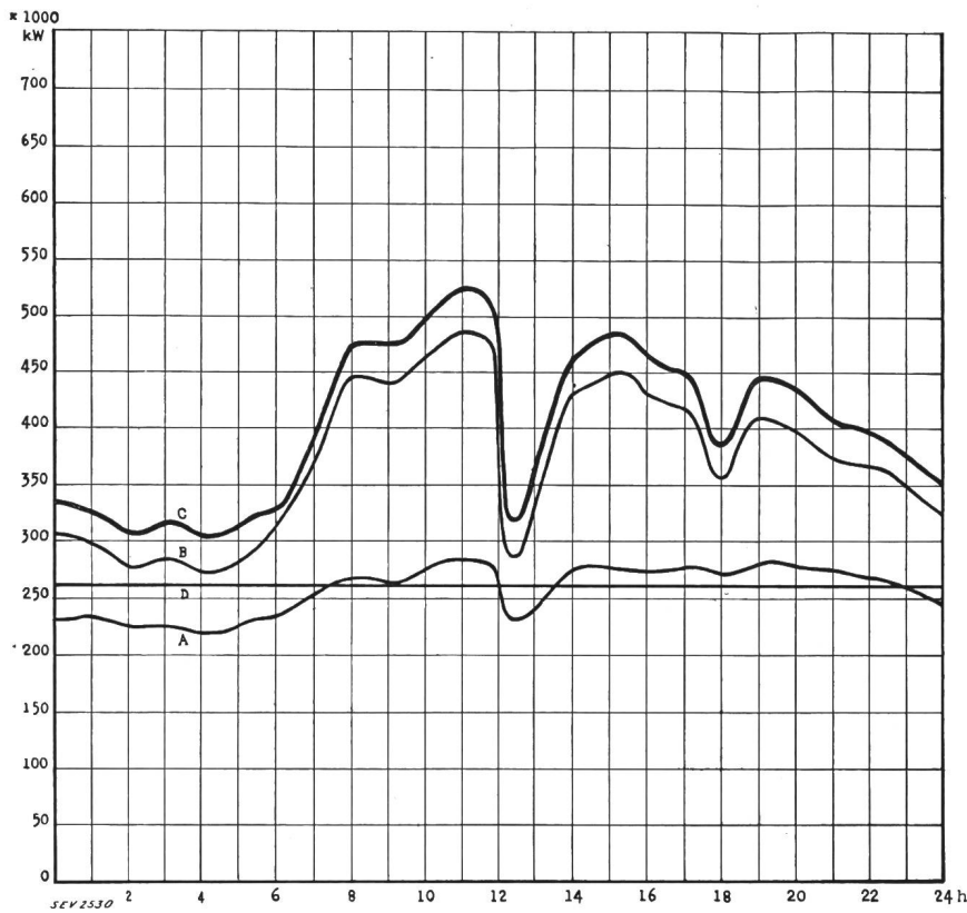
Diagramme journalier des puissances utilisées, mercredi le 16 mars 1932.
