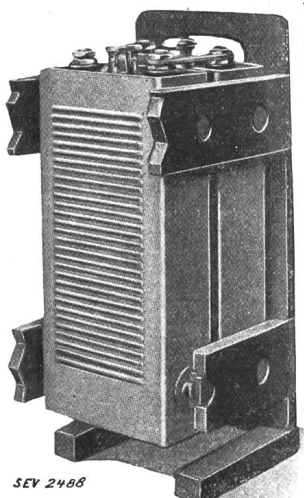
Fig. 2. Zusammenbau der Elemente zu tragbaren Batterien.
