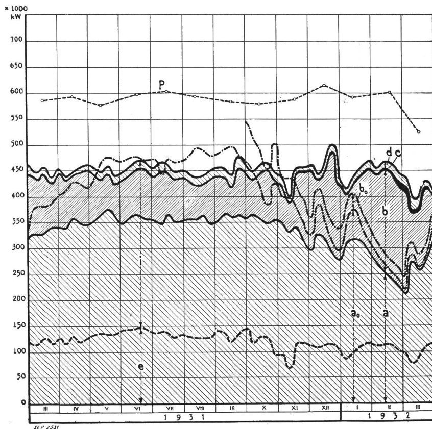
Diagramme annuel des puissances disponibles et utilisées, mars 1931 à mars 1932.
