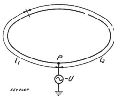
Fig. 8. Erdschluss im Punkt P einer Ringleitung.
