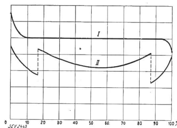
Fig. 12. Ölgefüllte Durchführungen für 187 kV. Verlauf der Achsial- und Radial-Gradienten. I Achsial. II Radial.
