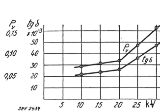
Fig. 1. Dielektrische Verluste P_v u. Verlustwinkel \operatorname{tg} \delta einer Mikanitisolation in Abhängigkeit der Spannung.
