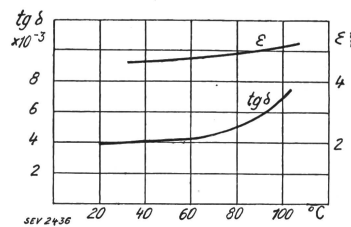
Fig. 3. Verlustwinkel \operatorname{tg} \delta und Dielektrizitätskonstante \epsilon in Abhängigkeit der Temperatur.
