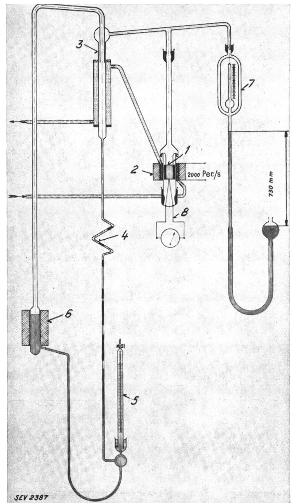
Fig. 1. Glasapparatur zur quantitativen Bestimmung der aus festen Materialien bei Erhitzung unter Vakuum austretenden Gase.
