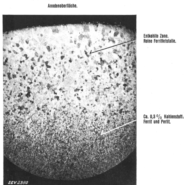
Fig. 4. Mikrophotographie eines Schliffes durch Anodeneisen. Vergrößerung 16 : 1.
