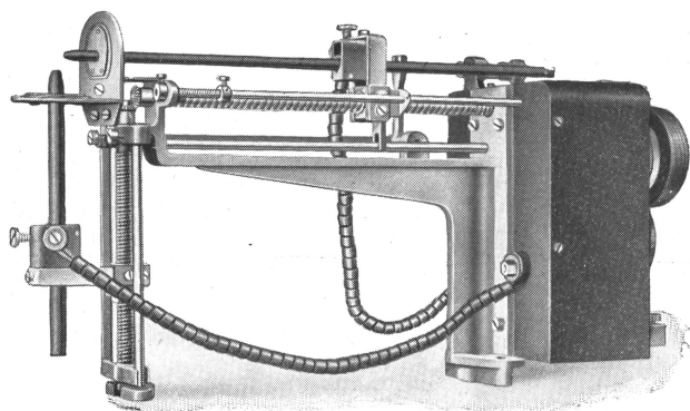
Fig. 6. Mikroprojektions-Bogenlampe.
