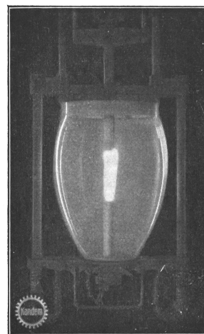
Fig. 5. Lichtbogen der Pauslampe, richtig brennend, falsch brennend.
