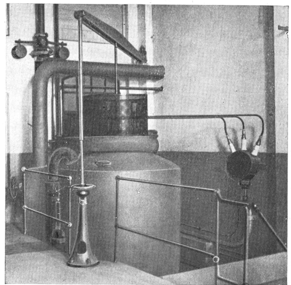
Fig. 2. Der 1923 in Attisholz aufgestellte Sulzer-Hochspannungselektrodendampfkessel, 5000 kW.
