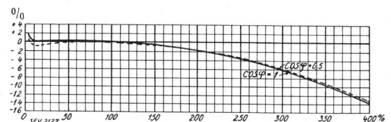
Fig. 1. Lastkurven eines Einphasenwechselstrom-Zweileiterzählers älterer Konstruktion. Prozentuale Fehler in Funktion der prozentualen Belastung.
