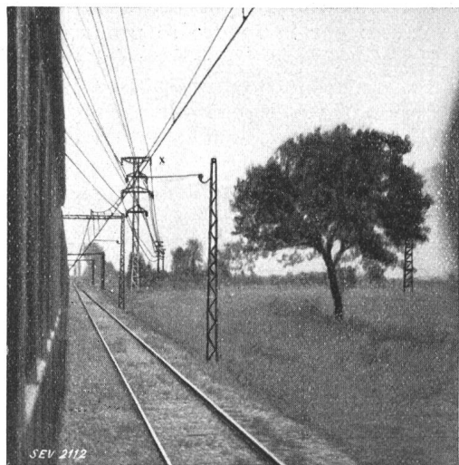
Fig. 12. Pylône du croisement dérangé, chap. III, 9.
