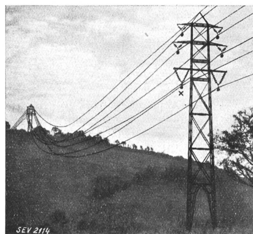
Fig. 14. Pylône n° 209 dérangé, chap. III, 11.
