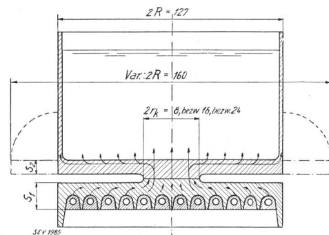
Fig. 3. Idealisiertes Drittel der Wärmeübertragung der 22 cm-Kochplatte auf Wasser als Kochgut.
