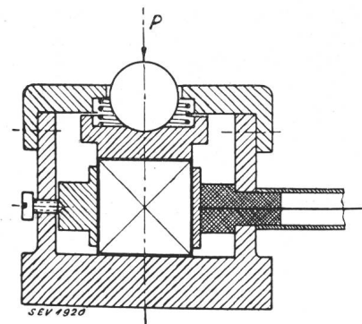
Fig. 11. Quarzdruckkammer des Messgerätes von Kluge und Linckh zur piezoelektrischen Messung von Druck- und Beschleunigungskräften (vergl. VDI 1929, 73, S. 1311).
