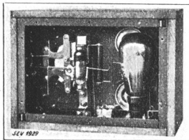
Fig. 20. Innenansicht des Verstärkers
