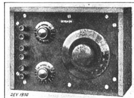
Fig. 21. Aussenansicht des Verstärkers
