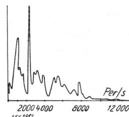
Fig. 8. Tonspektrum des Geräusches eines Staubsaugers (nach Grützmaier). Schalleistung in Funktion der Frequenz.
