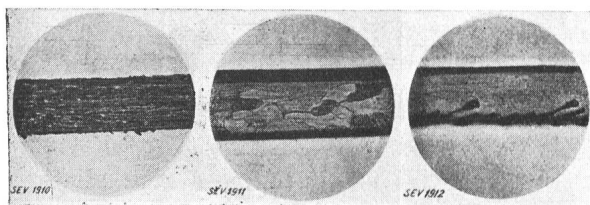
Fig. 1. Nach dem Hämmerverfahren hergestellter Wolframdraht (Ziehstruktur).
