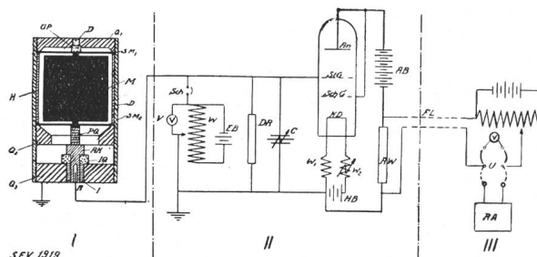
Fig. 10. Der registrierende Beschleunigungsmesser der «Prospektion» G. m. b. H. (Göttingen) nach dem Piezo-Quarzplattensystem. I Erschütterungsmesser. II Umformer und Eichungsvorrichtung. III Registrierapparat.
