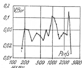
Fig. 6. Frequenzkurve eines normalen Fernsprechmikrophons.
