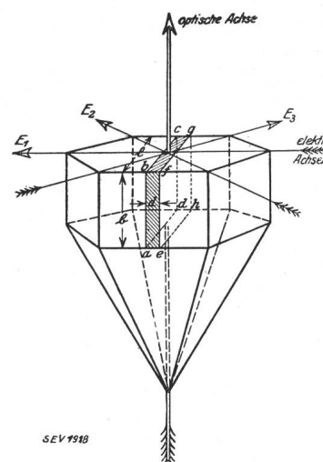
Fig. 9. Quarzkristall mit der optischen und den elektrischen Achsen.
