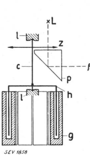
Fig. 5. Schematische Darstellung des Messwerkes.
