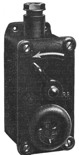
Fig. 3. Automatische Steckdose.
