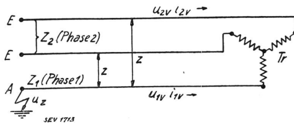
Fig. 34. Wellenschema der unverzweigten Drehstromleitung: \delta = z/Z ; \kappa = Z_2/Z_1 .
