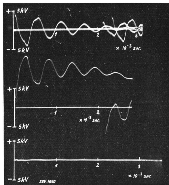
Fig. 11. ( f ) Versuchs-No.: 254-250-260. Messung in Phase 1: Leitungsseite des Induktionsreglers. Messung in Phase 3: Transformierseite des Induktionsreglers. Messung in Phase 1: Ueber den Induktionsregler.
