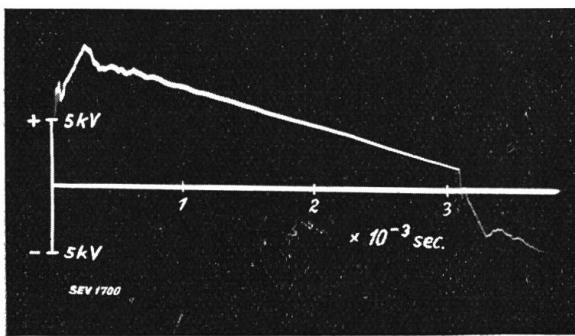
Fig. 21. (f) Versuchs-No.: 489; Messung in Phase: 2.
