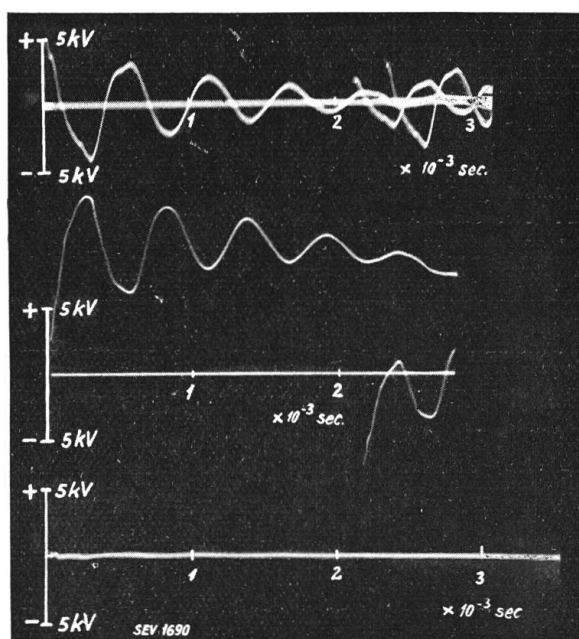
Fig. 11. ( f ) Versuchs-No.: 254–250–260. Messung in Phase 1: Leitungsseite des Induktionsreglers. Messung in Phase 3: Transformerseite des „ Messung in Phase 1: Ueber den Induktionsregler.
