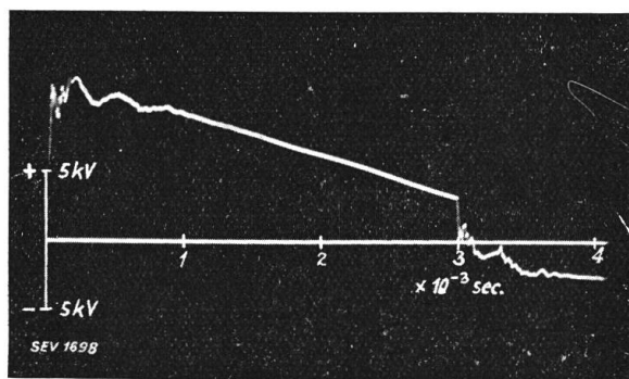
Fig. 19. (f) Versuchs-No.: 457; Messung in Phase: 2.
