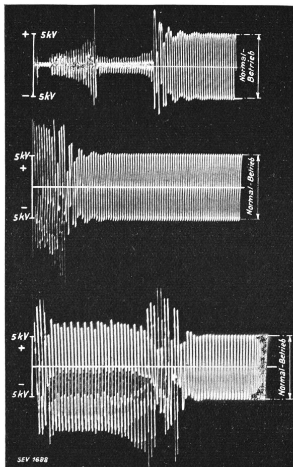
Fig. 9. ( i ) Versuchs-No. 154–156–167; Messung in Phasen: 1–2–2.
