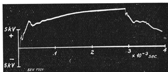
Fig. 22. (f) Versuchs-No.: 504; Messung in Phase: 3.
