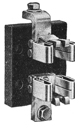
Fig. 7. Sicherungsunterteil 350 A für Einbau in Kabelverteilungs-schränke und Anschluss von Sammelschienen.
