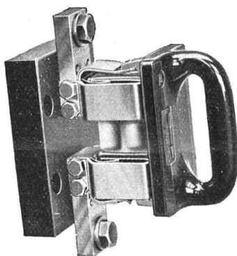
Fig. 5. Geschlossene Griff-sicherung.
