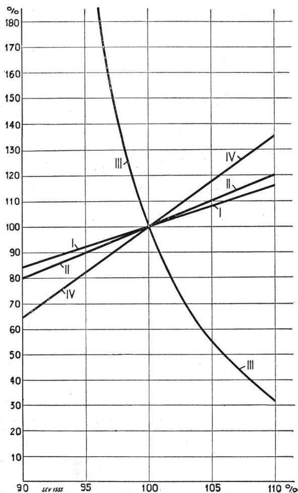
Fig. 1. Abscisses: Tension d'exploitation en % de la tension d'estampillage. Ordonnées: Courbe I Puissance absorbée (W) en % de la puissance normale. Courbe II Rendement lumineux (Lm/W) en % du rendement normal. Courbe III Longévité (h) en % de la longévité normale. Courbe IV Flux lumineux (Lm) en % du flux normal.
