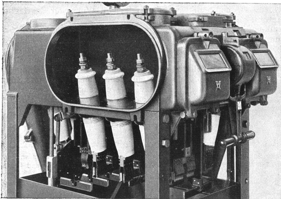
Fig. 12. Gussgekapelte Verteilung für 6 kV, 100 000 kVA.
