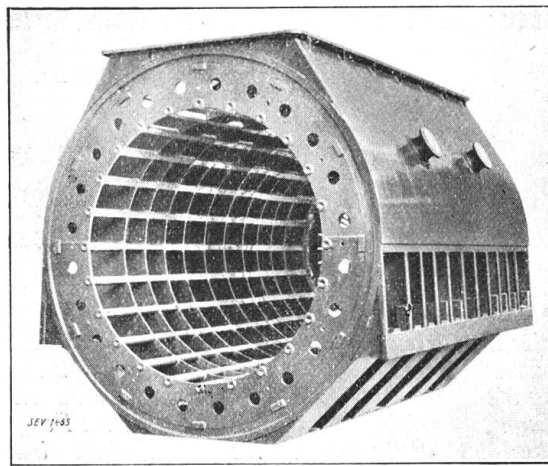
Fig. 21. Turbogehäuse für Generator, 45000 kVA, der A.-G. Brown, Boveri & Co.
