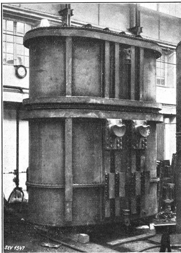
Fig. 4. Geschweisster Kessel für Grosstransformator der A.-G. Brown, Boveri & Co.
