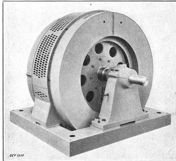
Fig. 14. Drehstrommotor, 1000 PS, der Maschinenfabrik Oerlikon.
