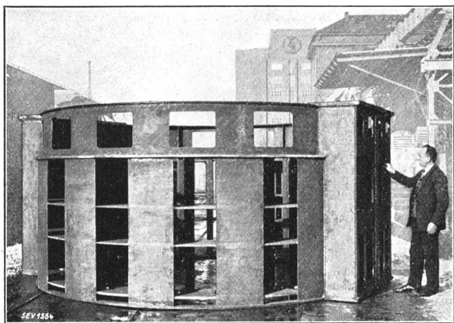
Fig. 20. Gehäuse für Vertikalgenerator, 27000 kVA, der Siemens-Schuckert-Werke.
