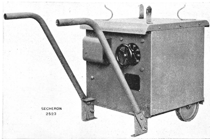
Fig. 3. Schweisstransformator der S. A. des Ateliers de Sécheron.
