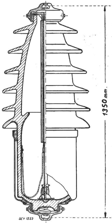
Fig. 1. Porzellankondensator.
