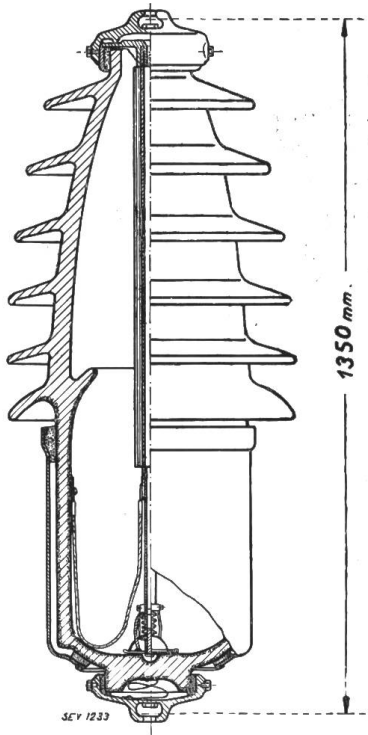
Fig. 1. Porzellankondensator.
