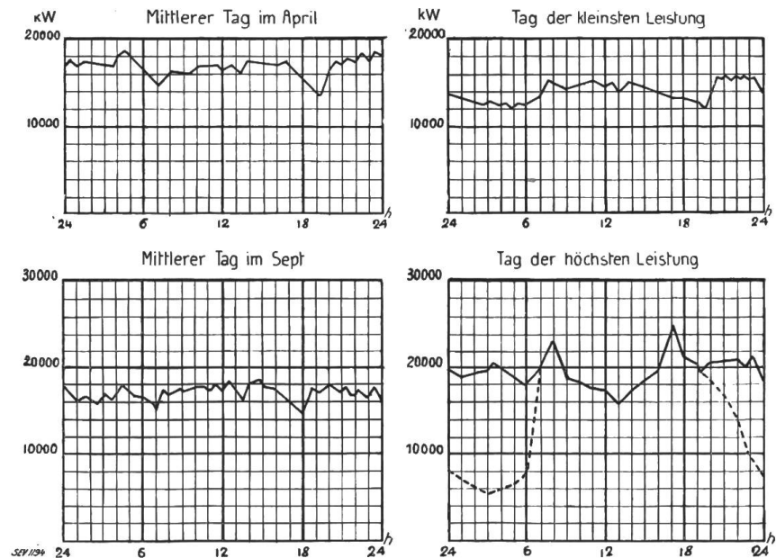
Fig. 5. Tagesleistungskurven 1928.
