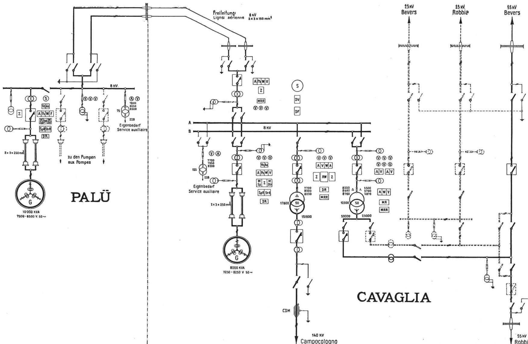
Fig. 10. Kraftwerke Palù-Cavaglia. Schaltungsschema.
