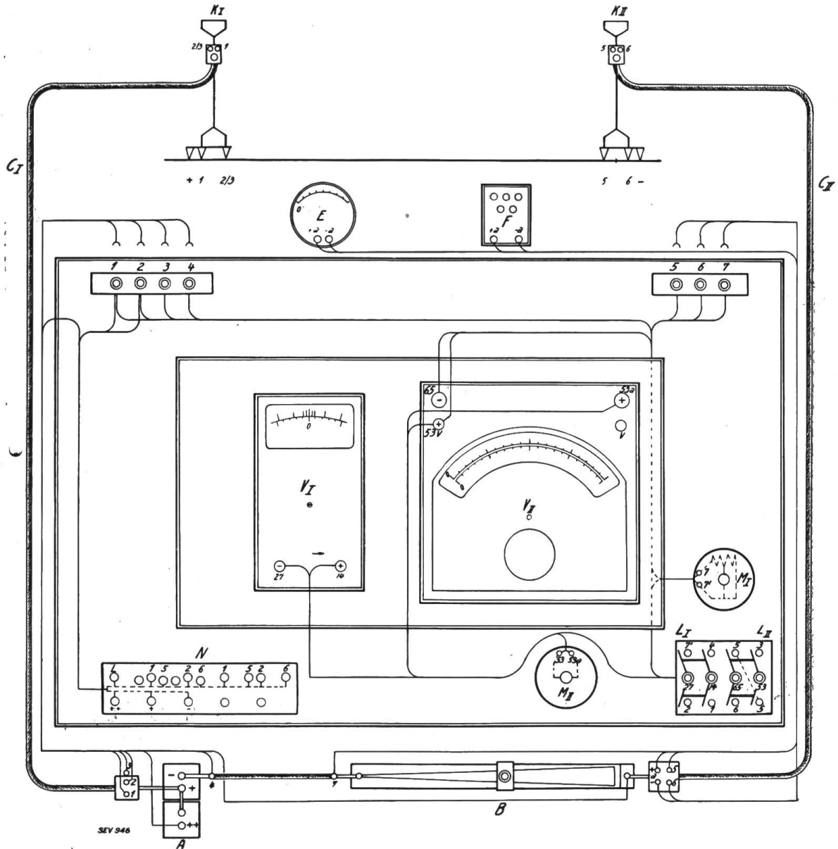
Fig. 4. Schéma détaillé.
