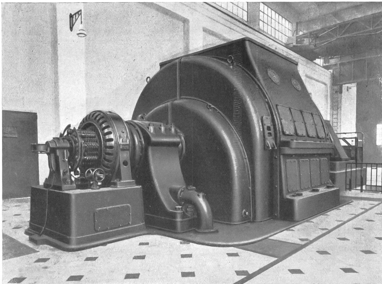
Fig. 5. Versuchsmaschinengruppe.
