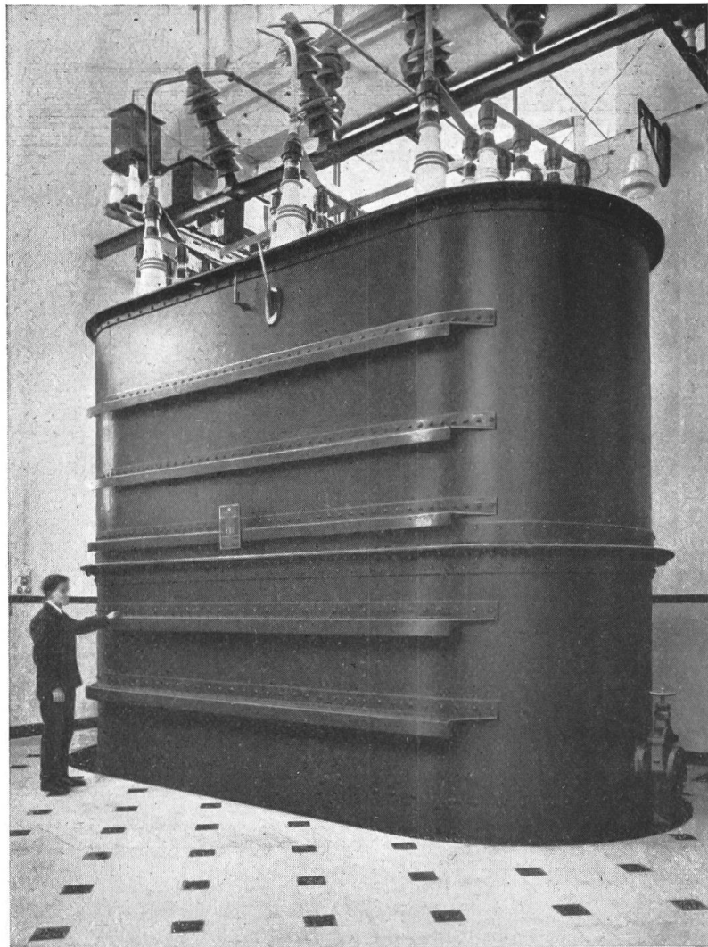
Fig. 6. Hochspannungstransformator.
