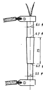
Fig. 11. Cône d'acier avec thermo-élément, pour l'épreuve de résistance au feu.
