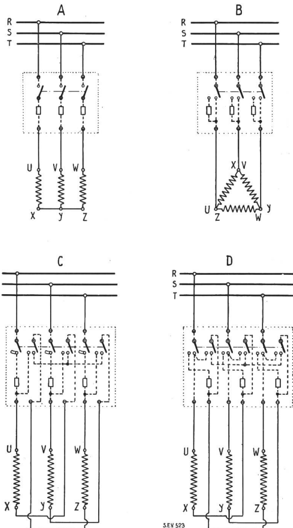
Schémas de connexions pour interrupteurs sous coffret
