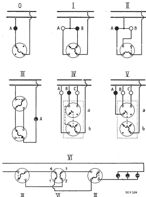
Schémas de connexions pour interrupteurs sous boîte.
