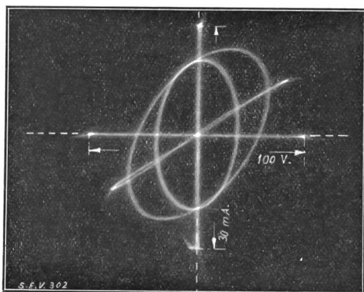
Fig. 28. Beispiel eines an Stromwandler No. 3 aufgenommenen Impedanz-Oscillogramms, samt zugehörigen Eichwerten für Spannungs- und Stromachse.
