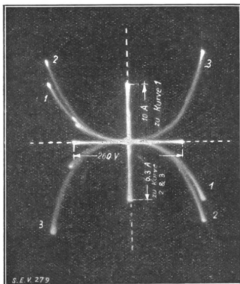
Fig. 14. Widerstands-Oscillogramme eines Silittringes mit 200 \Omega Nennwert, samt Eichwerten der Spannungs- und Stromachse. Kurven 1 bis 3: Drei Aufnahmen bei annähernd derselben Spannung. Für Kurve 3 Anschluss der Spannungs-Ablenkplatten vertauscht.
