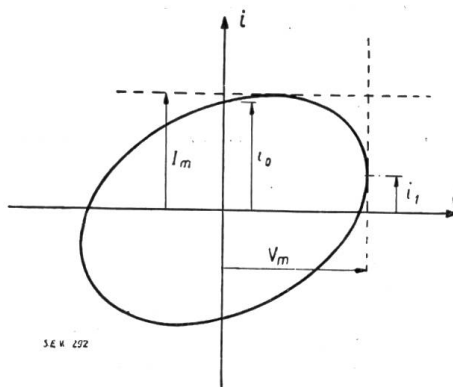
Fig. 27. Erklärung des Impedanz-Oscillogramms.
