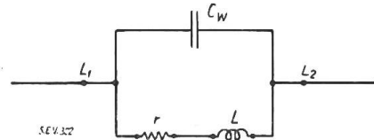
Fig. 37. Durch die Versuche erwiesenes Ersatzschema für das Verhalten des Stromwandlers bei Hochfrequenz.
