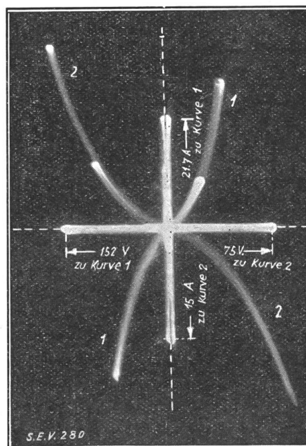
Fig. 15. Widerstands-Oscillogramme eines Silittringes mit 5 \Omega Nennwert, samt Eichwerten der Spannungs- und Stromachse. Anschluss der Spannungs-Ablenkplatten zwischen den Aufnahmen 1 und 2 vertauscht.
