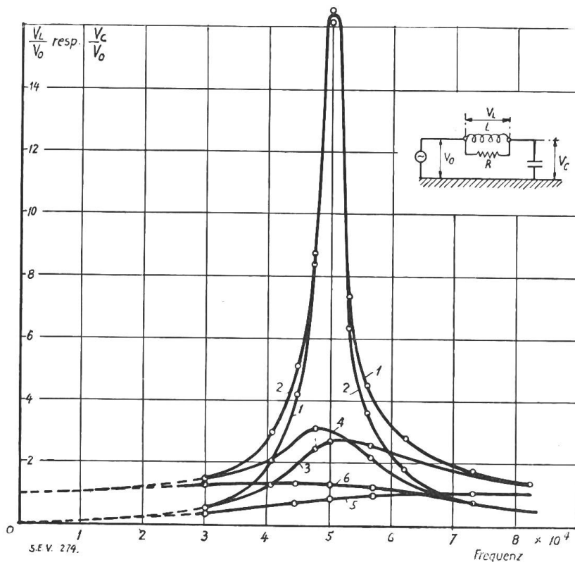
Fig. 9. Resonanzkurven für Stromwandler No. 3 mit einer ca. 100 m Kabel entsprechenden Kapazität, Eigenfrequenz 50 000 Perioden.
