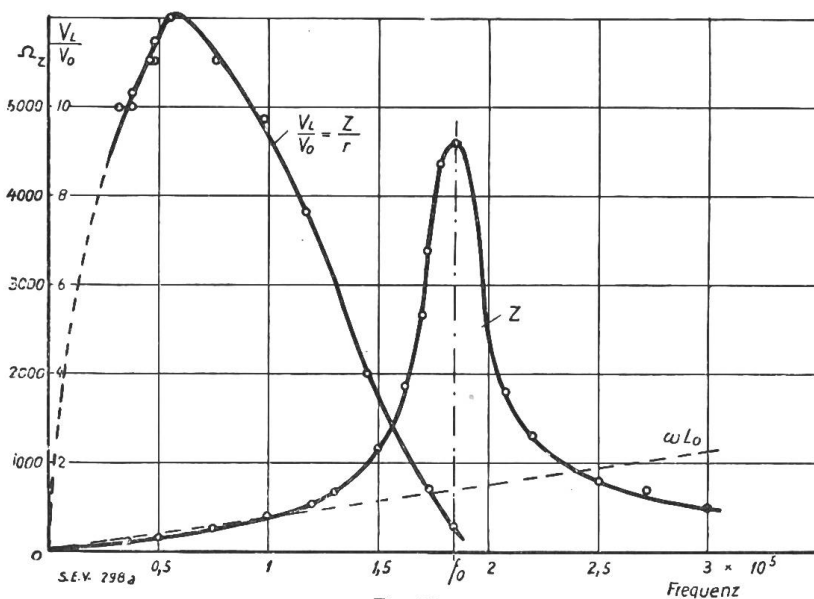
Fig. 33a. Impedanzkurve Z und Resonanzspannungskurve \frac{V_L}{V_0} für Stromwandler No. 4, Schaltung 25/5 A, im Frequenzbereich bis 3 \times 10^5 Perioden. Bedeutung von \omega L_0 siehe Fig. 32a.
