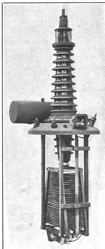
Fig. 14. Widerstand, aus dem Oelkübel herausgenommen.
