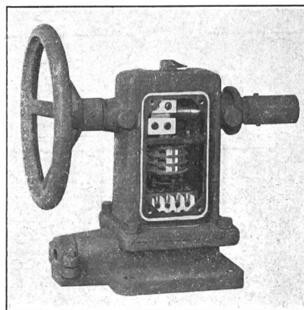
Fig. 11. Handradantrieb eines dreipoligen Drehtrennmessers.
