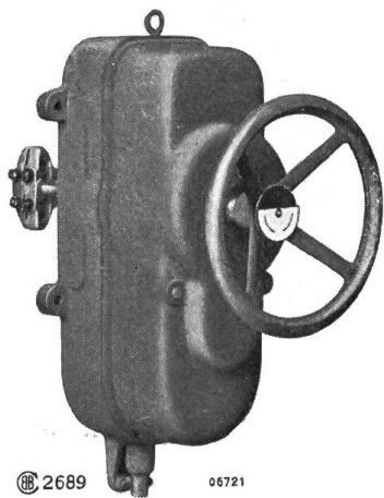
Fig. 6. BBC - Motorferntrieb.
