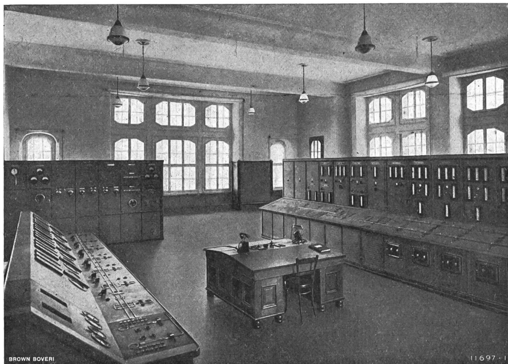
Fig. 10. Kommandoraum des Kraftwerkes Gösgen.
