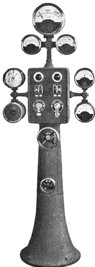
Fig. 1. Schaltsäule.
