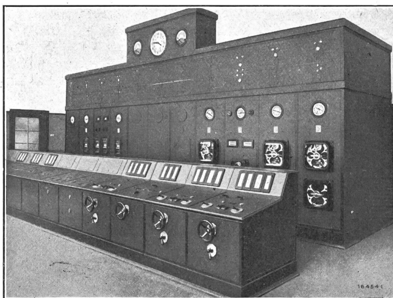
Fig. 11. Kommandoraum des Kraftwerkes Barberine der Schweiz. Bundesbahnen.
