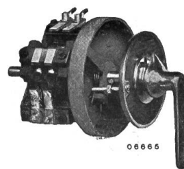
Fig. 7. BBC - Steuerschalter oder Kontaktgeber.
