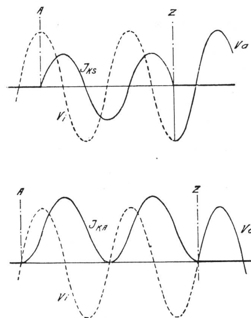
Fig. 1. Symmetrischer und asymmetrischer Verlauf des Kurzschlussstromes.
